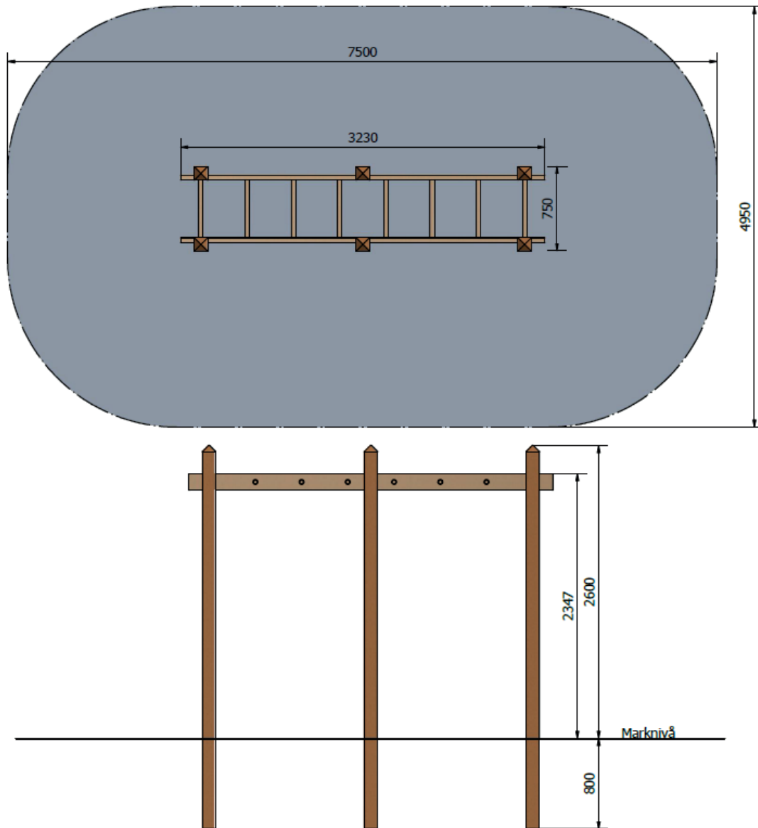
Vy ovanifrån med säkerhetsområde samt vy från sidan (mm)
