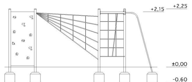
Vy från sidan med höjder/djup (m)
