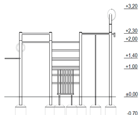
Vy från sidan med höjder/djup (m)
