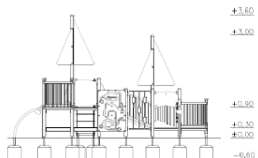
Vy från sidan med höjder/djup (m)
