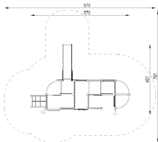
Vy ovanifrån med fallutrymme (cm)
