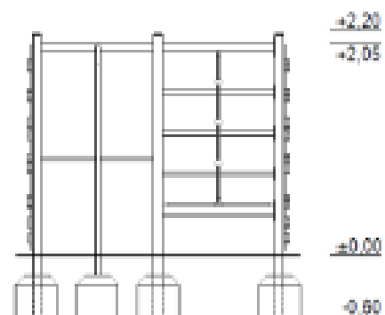
Vy från sidan med höjder/djup (m)
