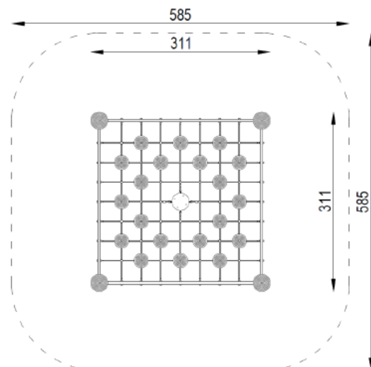
Vy ovanifrån med fallutrymme (cm)
