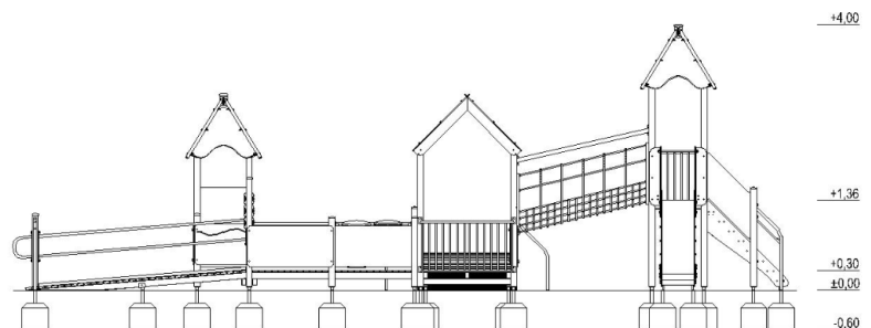
Vy från sidan med höjder/djup (m)
