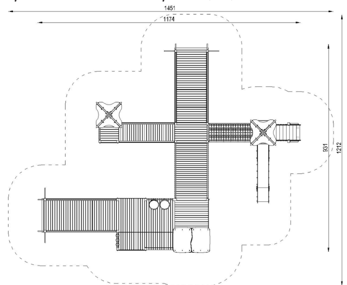
Vy ovanifrån med fallutrymme (cm)
