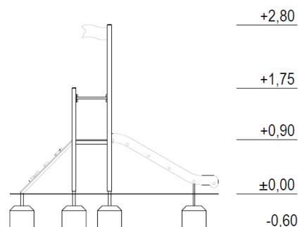
Vy från sidan med höjder/djup (m)
